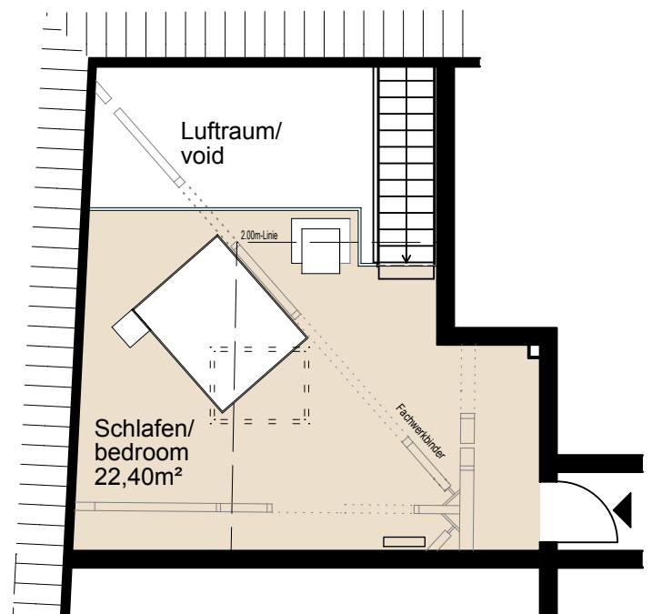
Dachgeschoss/ top floor
